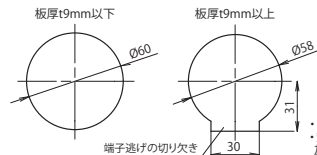
P650K / バッフル穴寸法図
