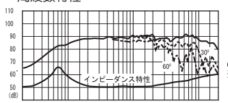
周波数特性
