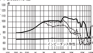
周波数特性
