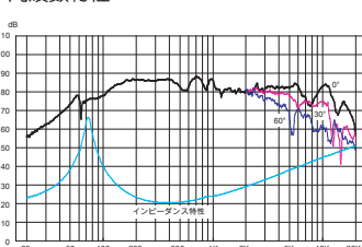
周波数特性
