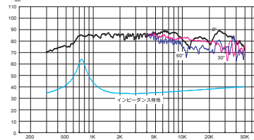
周波数特性
