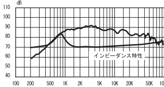
周波数特性
