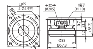
P650K / バッフル穴寸法図
