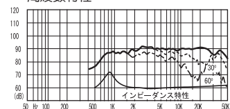
周波数特性
