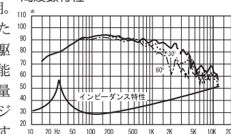
周波数特性
