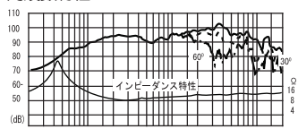
周波数特性
