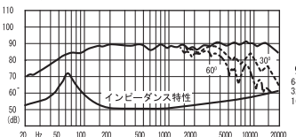
周波数特性
