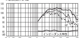
周波数特性
