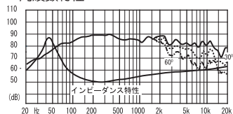
周波数特性
