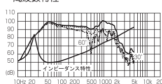
周波数特性
