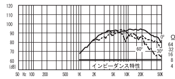
周波数特性
