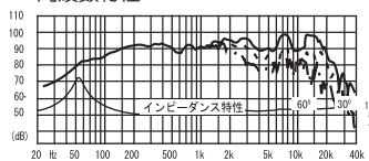
周波数特性
