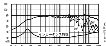
周波数特性
