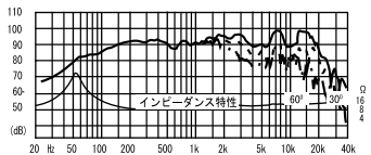
周波数特性
