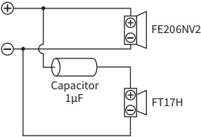
FE206NV2 + FT17H
