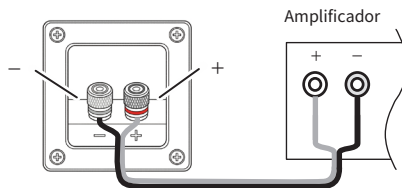
Seção do terminal
