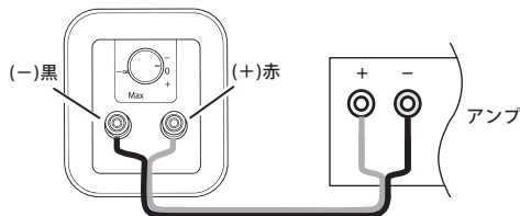
本体裏面ターミナル部
