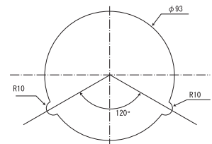
■バツフル開口寸法
