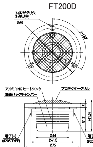
■バツフル取付寸法図
