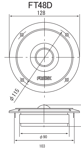
■バツフル開口寸法
