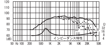
周波数特性
