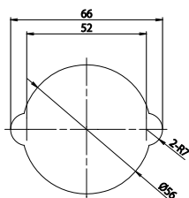
■バツフル取付寸法図
