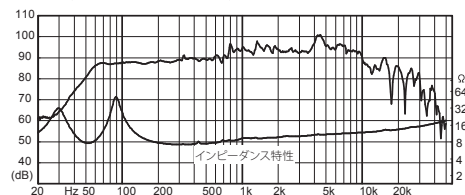
BK225WK (FF225WK 取り付け時)
