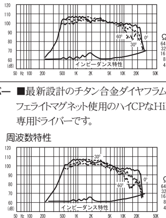
周波数特性
