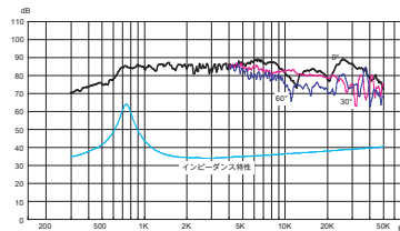
周波数特性
