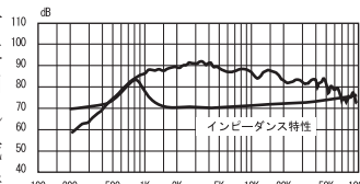
周波数特性
