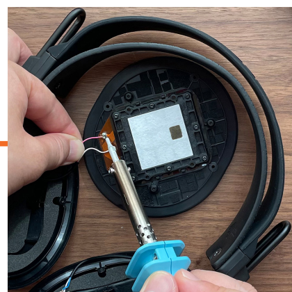
方式を選択するハウジング用チューニングシートの選択・取り付け、RP ドライバーユニットのはんだ付け
