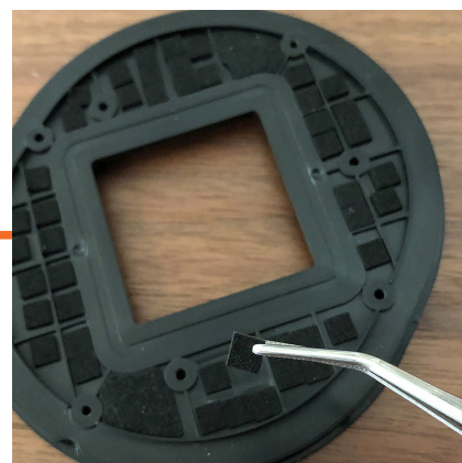
ハウジング用吸音材、バッフル用制振兼吸音材の取り付け
