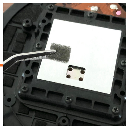
RP ドライバー・ユニットの取付、専用チューニング・ダンパーの取り付け
